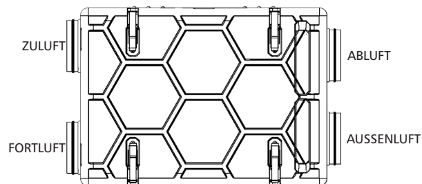
Abb. 16 – Anordnung der Anschlussstutzen für die Ausführungen L und LS
