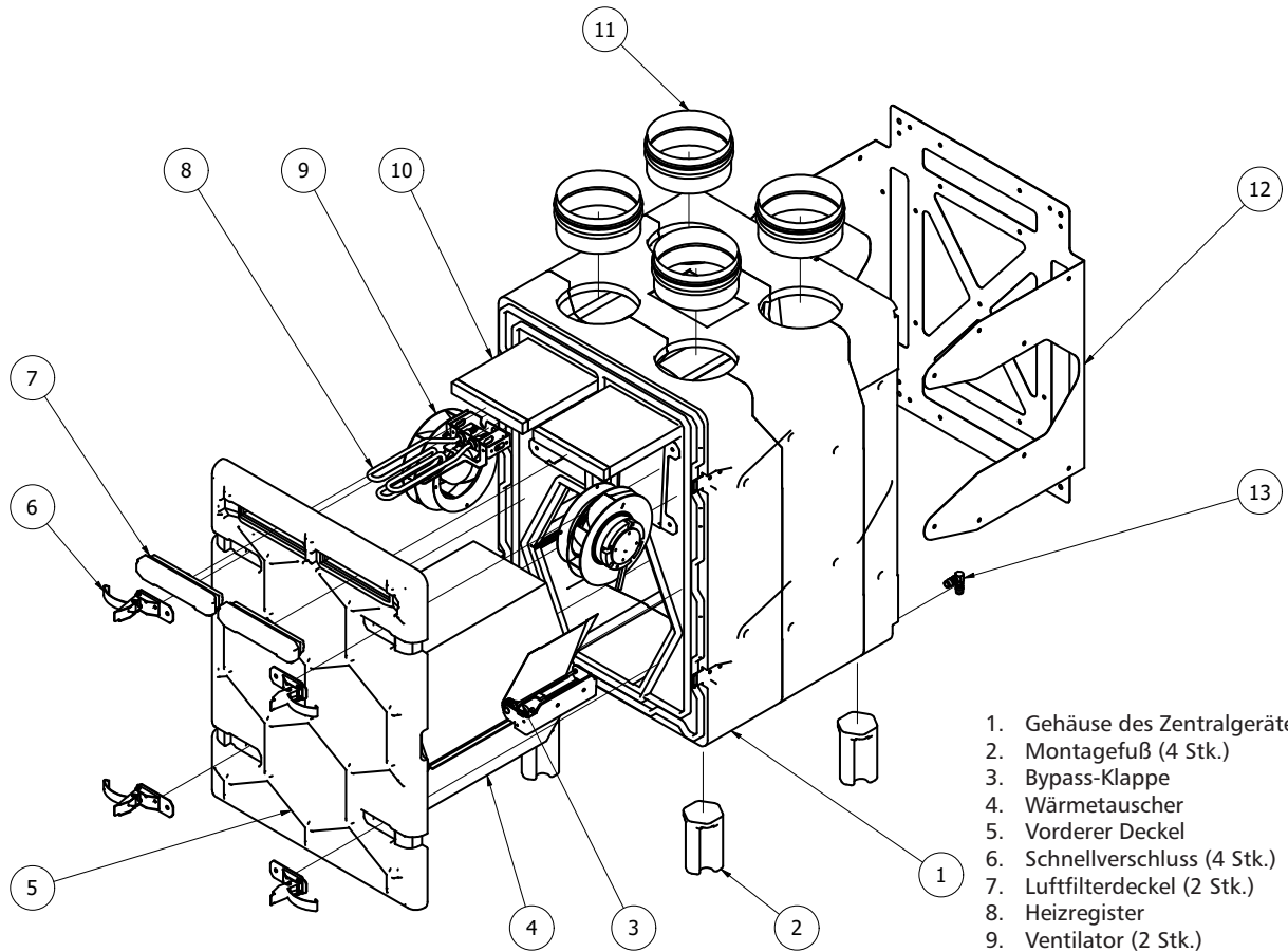
Abb. 2 – Konstruktionschema
