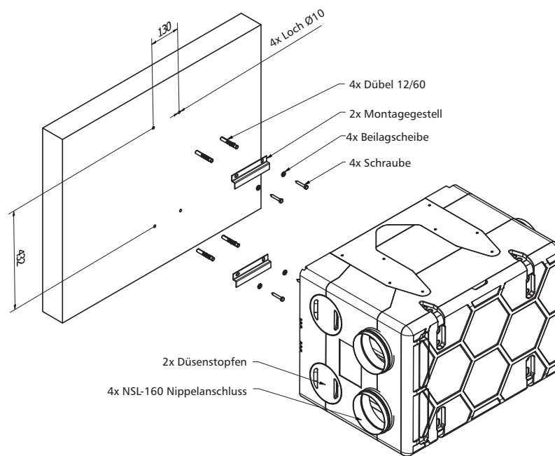
Abb. 10 – Montage mittels Montagegerahmen
