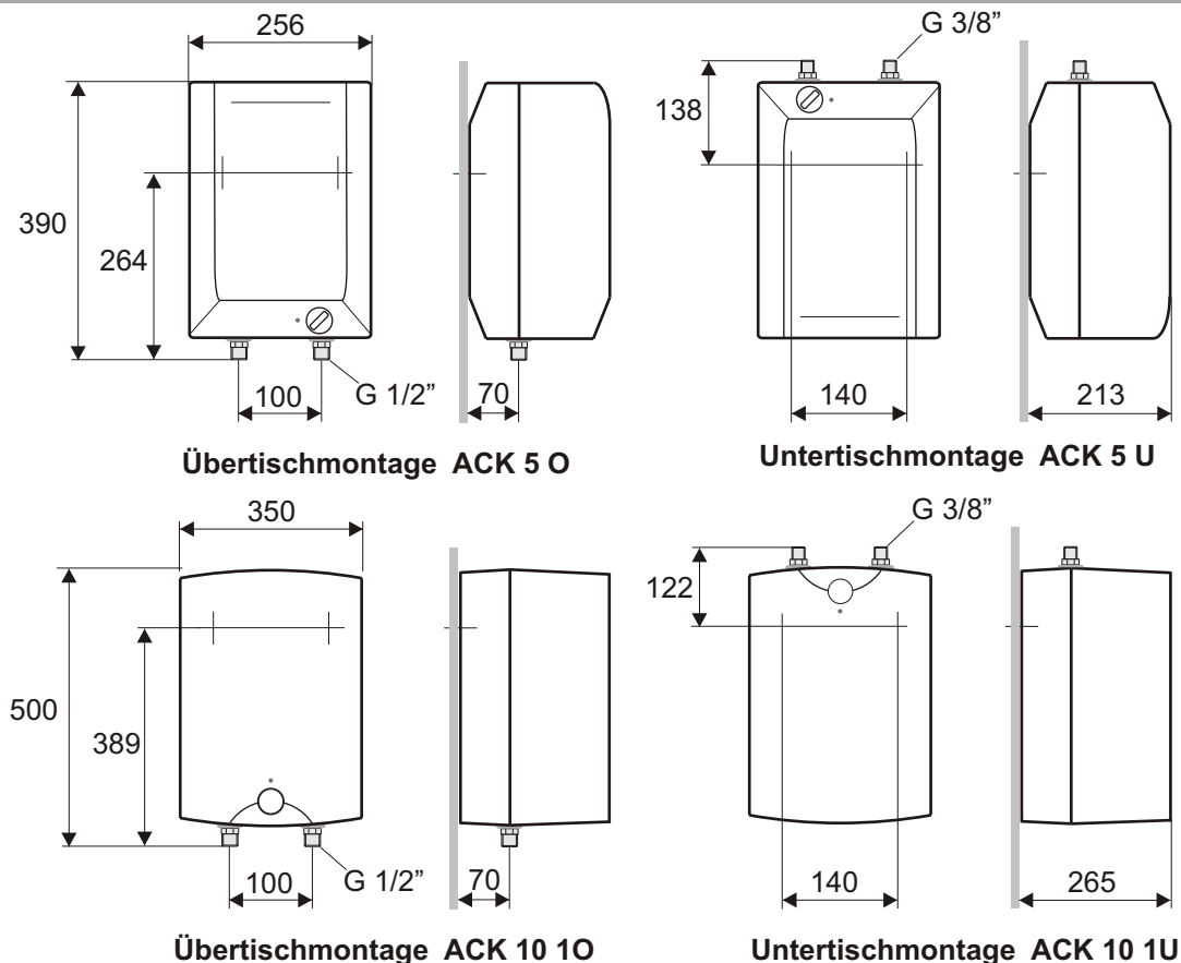
Bild 1: Geräteabmessungen und Montagemaße
