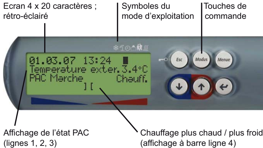
Fig. 4.1: Affichage standard sur écran à cristaux liquides, affichage principal avec touches de commande
