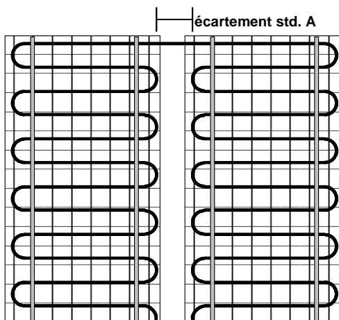
Ecartement entre les câbles chauffants
