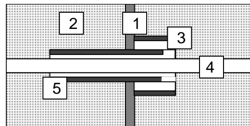
Pose d'extrémité froide à travers un joint de dilatation
