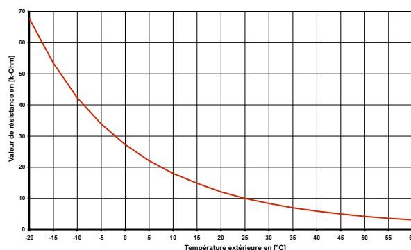
Fig. 7.1 : Courbe caractéristique de la sonde NTC-10 I
